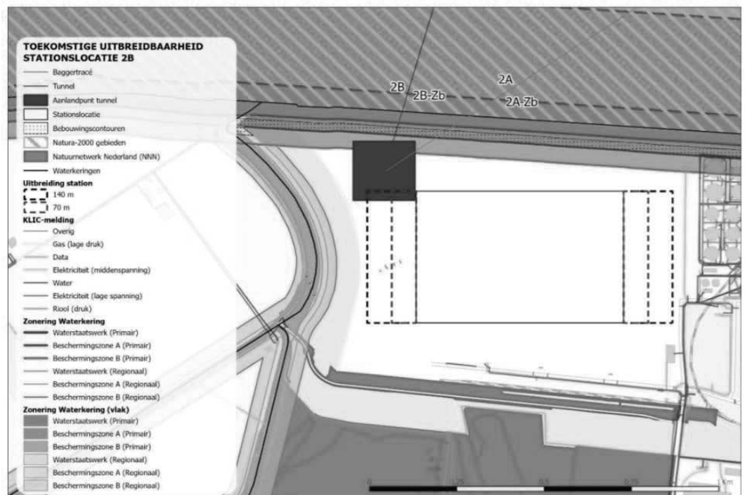
Figuur 7-5 Toekomstige uitbreidbaarheid integrale alternatieven met stationslocatie 2b
