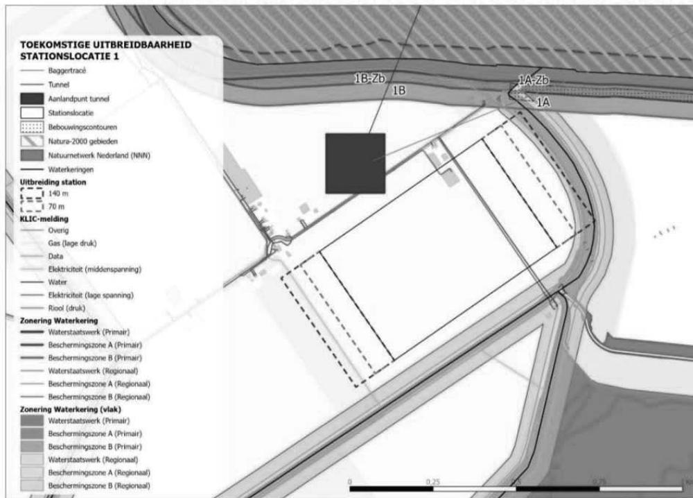
Figuur 7-4 Toekomstige uitbreidbaarheid integrale alternatieven met stationslocatie 1
